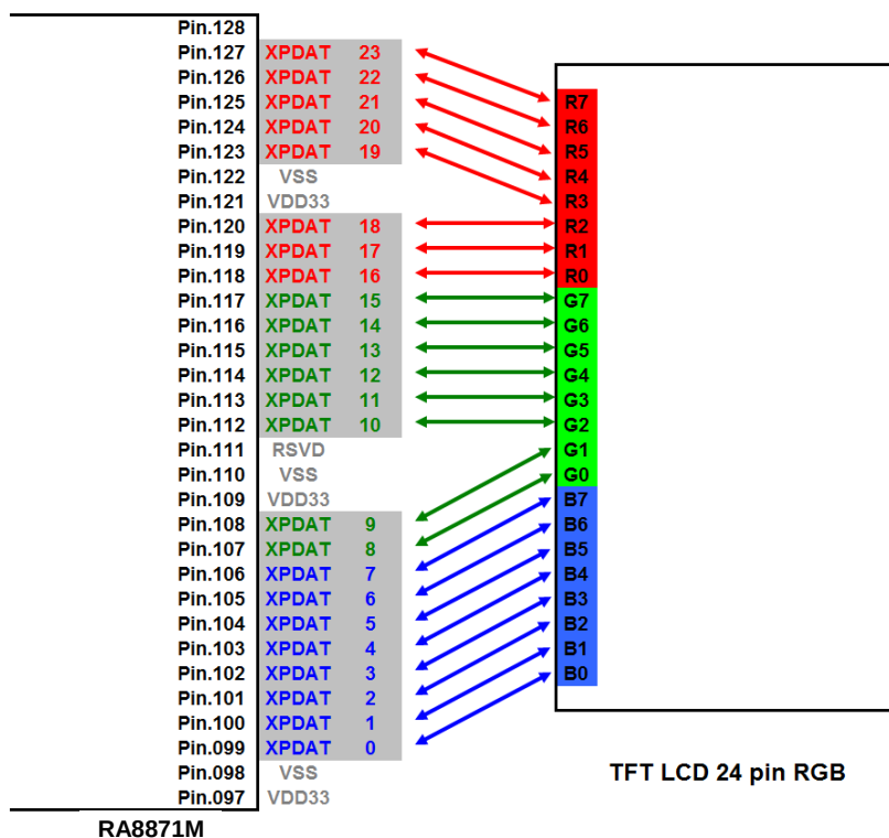
Figure 10-1 : RA8871M 色深 24bit 腳位與 LCD 螢幕腳位對應
