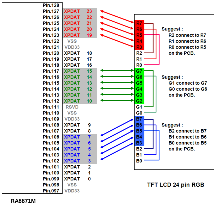
Figure 10-3 : RA8871M 色深 16bit 腳位與 LCD 螢幕腳位對應
