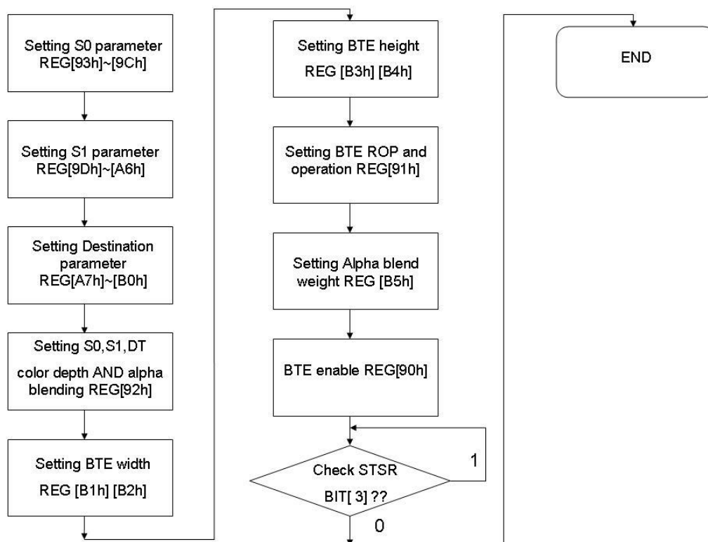
圖 13-30 : Picture Mode Flow Chart
