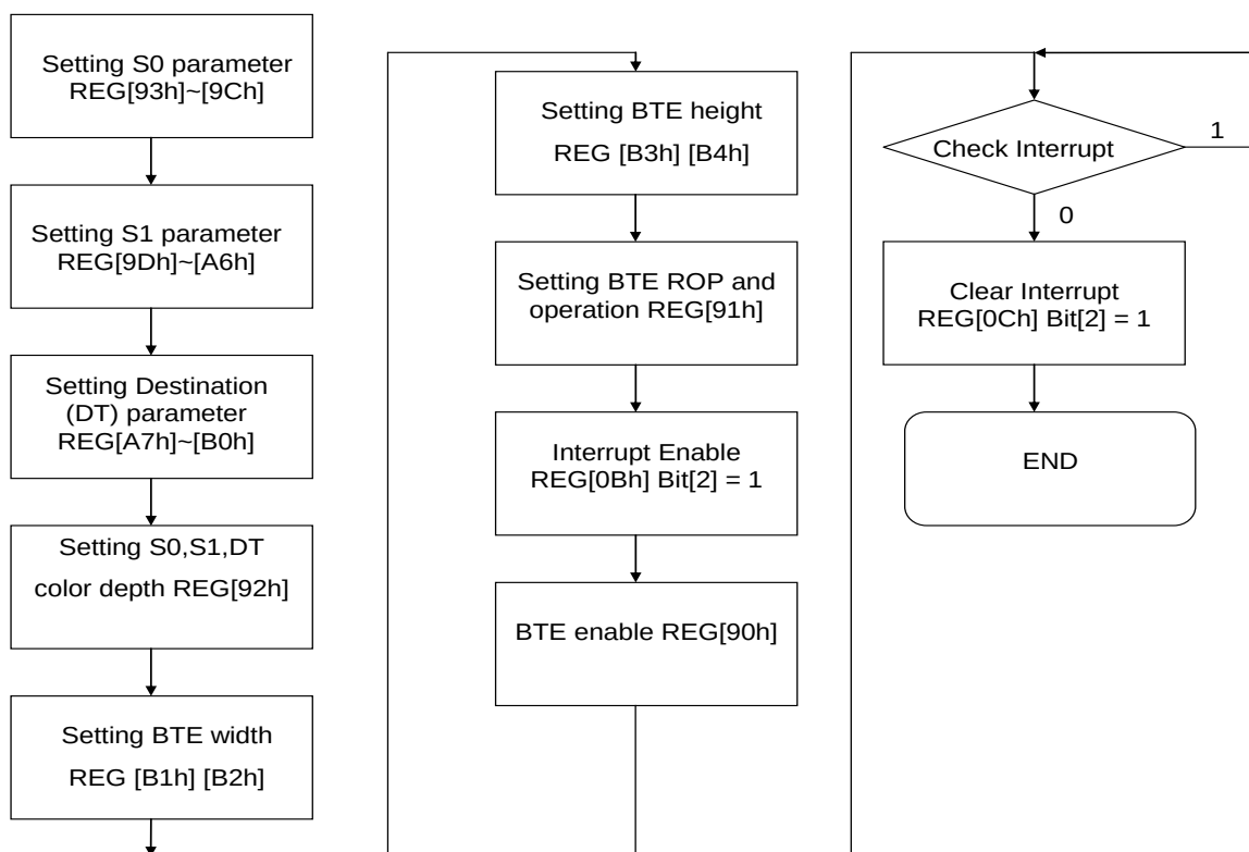
圖 13-9 : Flow Chart – Check Int
