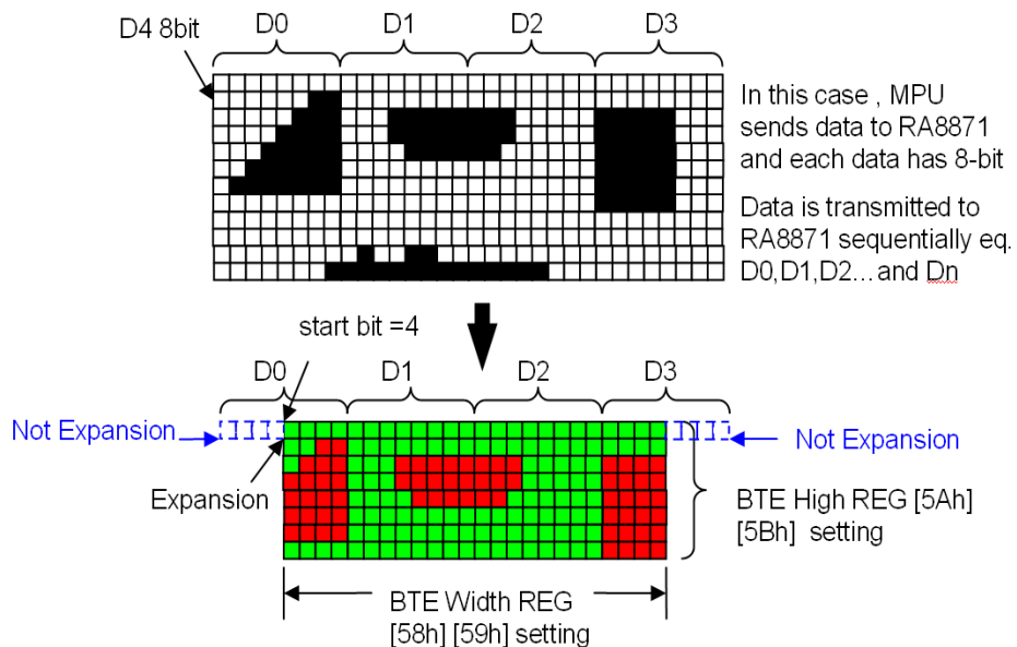
圖 13-23 : Color Expansion Data Diagram
