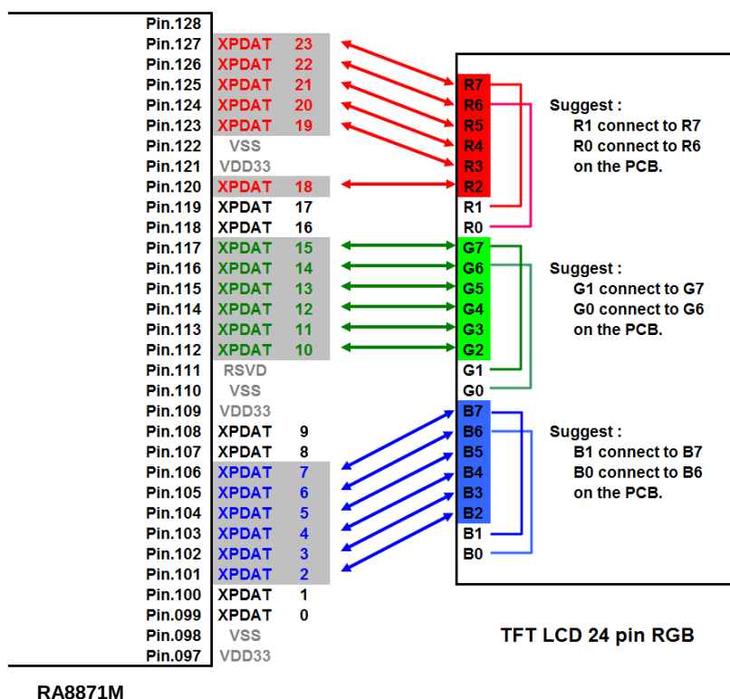
Figure 10-2 : RA8871M 色深 18bit 腳位與 LCD 螢幕腳位對應
