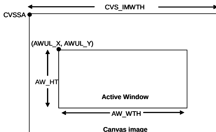
圖 19-4 : Active Window
