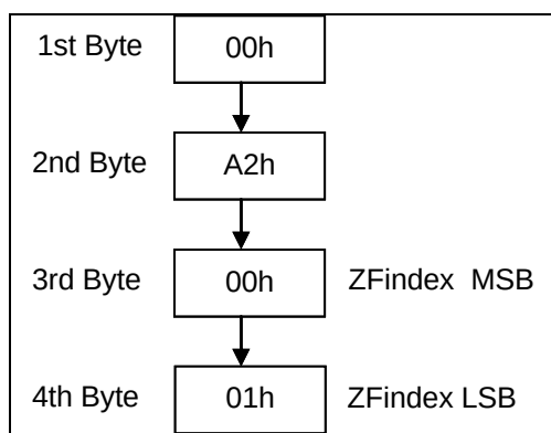
圖 16-9 : Uni-Code Zfindex
