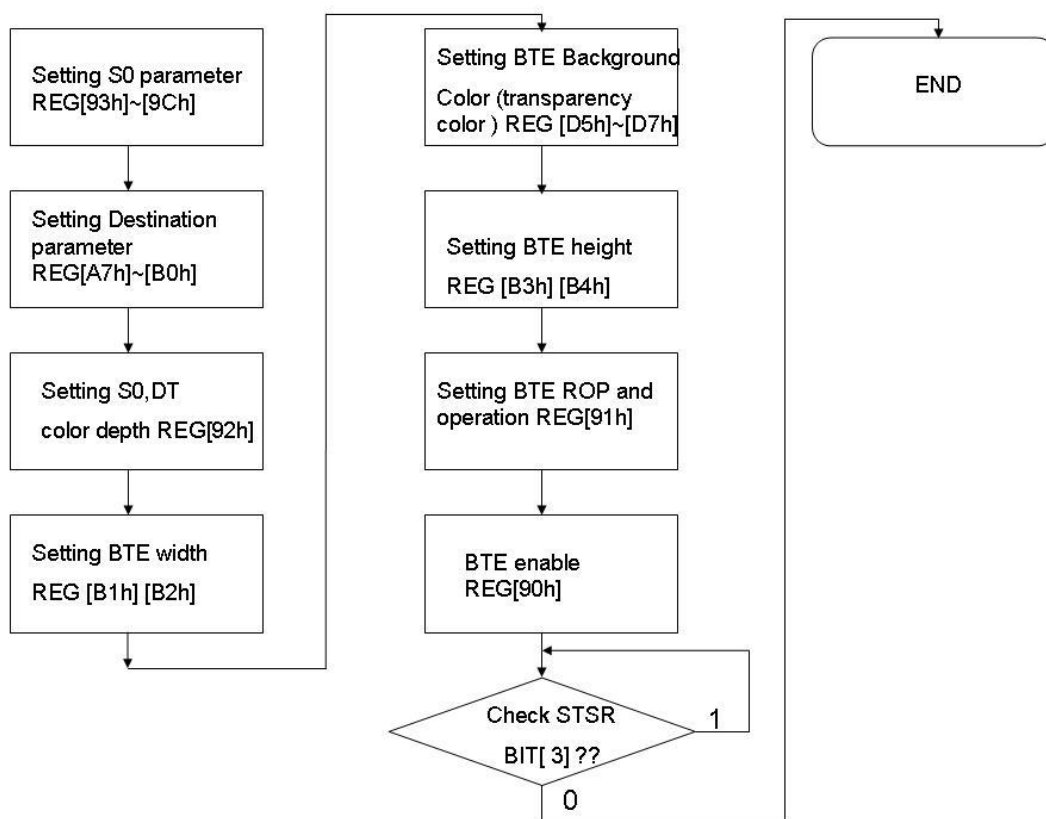
圖 13-12 : Flow Chart
