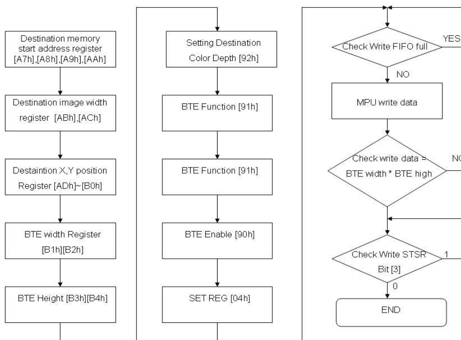
圖 13-25 : Flow Chart
