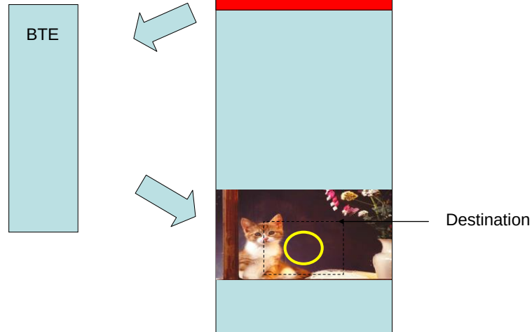
圖 13-13 : Hardware Data Flow
