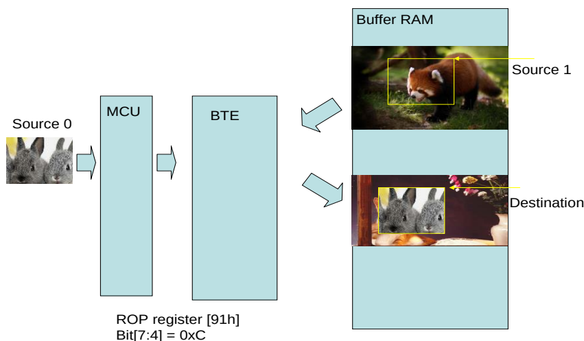
圖 13-5 : Hardware Data Flow
