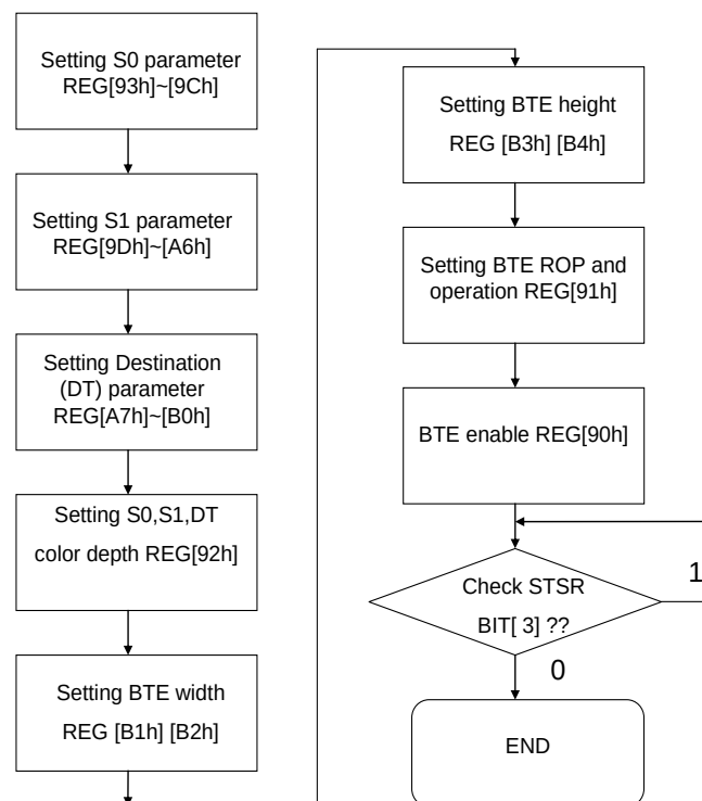
圖 13-8 : Flow Chart
