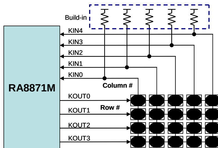
圖 17-1 : Key-Pad Application
